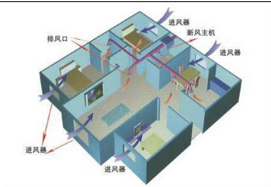
图 4.4-2 新风系统原理示意图
