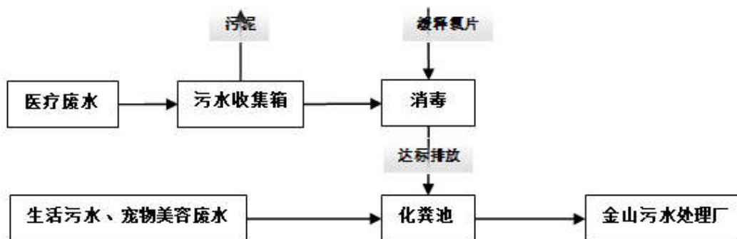
图 4.4-1 本项目废水处理工艺流程
